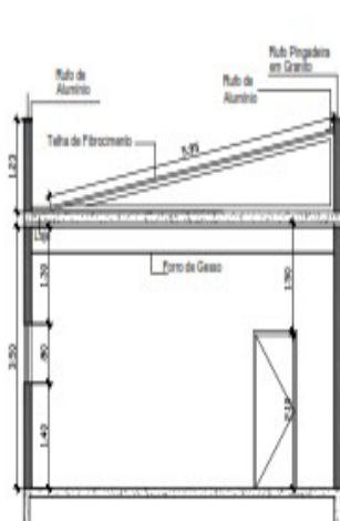
4 CORTE AA ESC: 1/50
